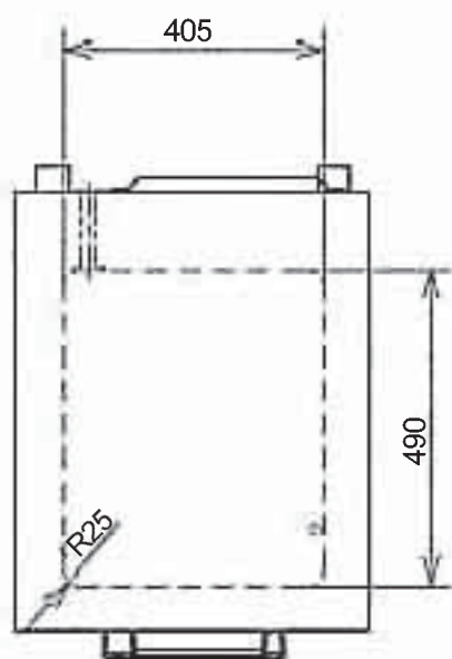
Top
