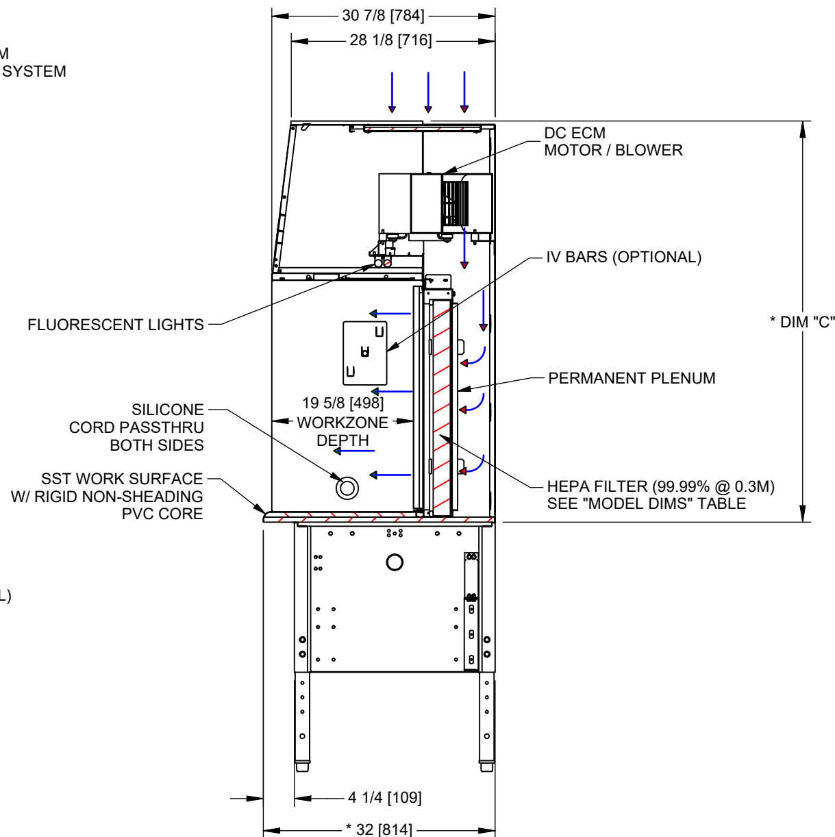
SECTION A-A
